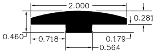
T-Molding (HTMLD)
